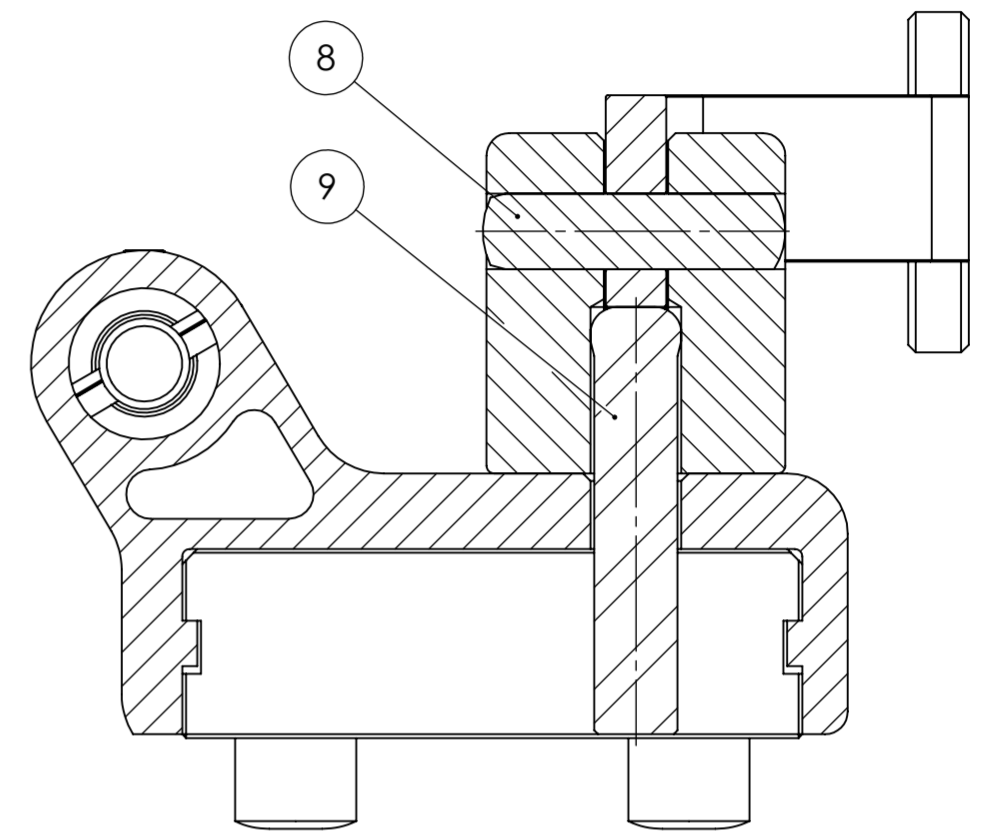
SCHNITT B-B
